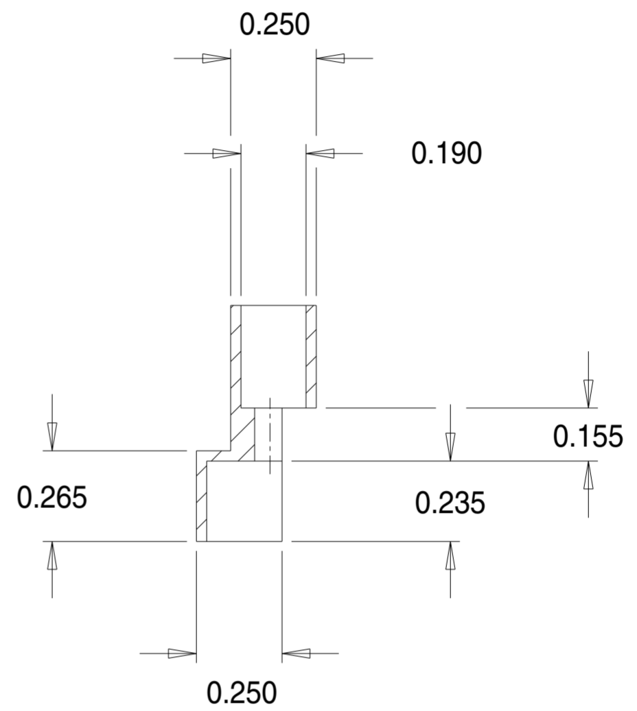
SECTION A-A
